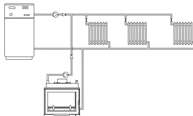
Exemple de principe si couplage avec une chaudière fioul, gaz ou électricité sur une installation existante. Raccordement chauffage en 33 x 42.
