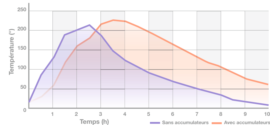
Comparaison de la température de l'air diffusé par l'appareil dans le temps avec ou sans accumulateurs.
