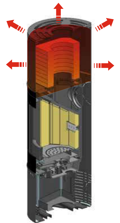
Accumulateur de chaleur réf. 965239 (en option sur certains appareils)
